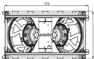
Μπροστά όψη
